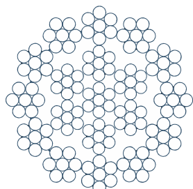
19x7 1+6
