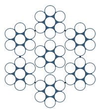
6 x 7 + AA 1 + 6
