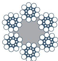
6 x 19 + AF Seale 1-9-9
