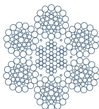
6 x36WS-AA CI WS 1-7-7+7-14
