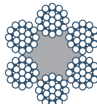
6 x 25 + AF Filler 1-6-6F-12
