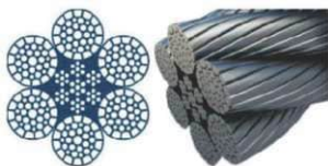
Compactado 6 pernas +AACI
