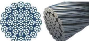
Compactado 35(34)x7
