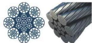
Compactado 8 pernas +AACI
