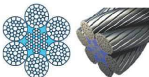
Compactado 6 pernas +AACI Revestida
