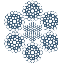
6 x41WS-AA CI WS 1-8-8+8-16
