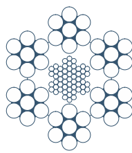
6 x 7 + AACI 1 + 6
